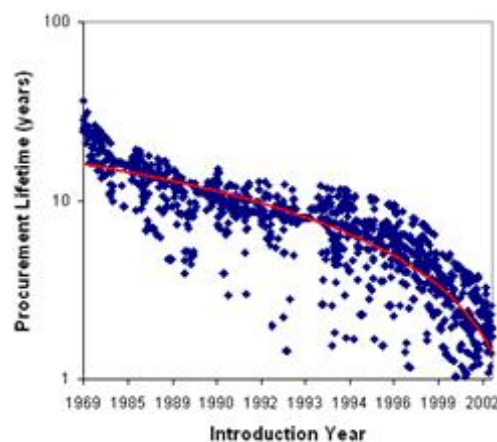
Fig. 3: Decrecimiento del tiempo de vida de los amplificadores operacionales, un componente existente en prácticamente toda aplicación electrónica
