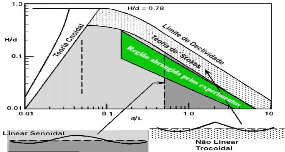
Figura 3 - Ilustração da região abrangida pelos ensaios
