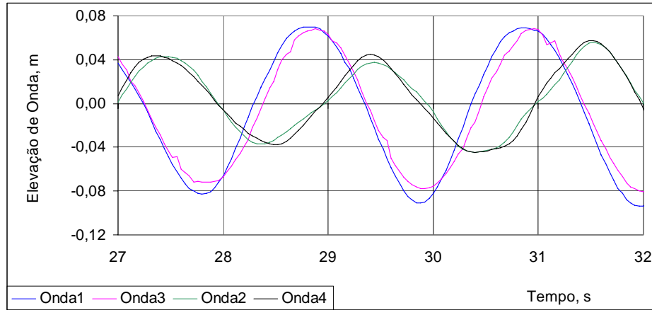
Figura 6 – Amostra de registro obtido de sinais dos medidores de onda ao longo do tanque.
