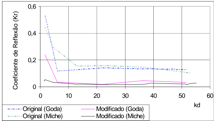
Figura 7 – Coeficientes de Reflexão nas duas configurações, medidos pelos métodos Miche (equação 12), e Goda e Suzuki.
