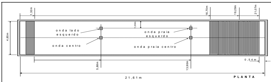
Figura 1 - Croquis das configurações do absorvedor de energia de onda.
