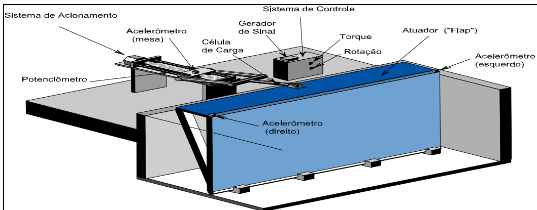
Figura 2 - Esquema e posições da instrumentação utilizada.
