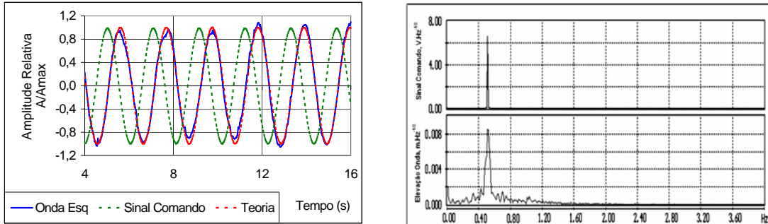
Figura 4 – Gráficos da comparação entre elevações de onda medida e calculada no tempo e dos espectros RMS dos sinais de comando e da elevação de onda, para f=0,5 Hz
