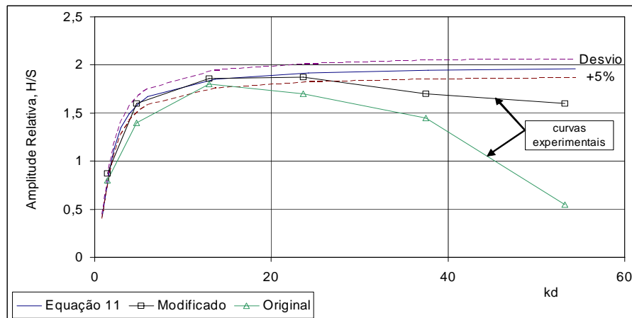
Figura 5 – Funções de Transferência do tanque, teórica e experimentais.
