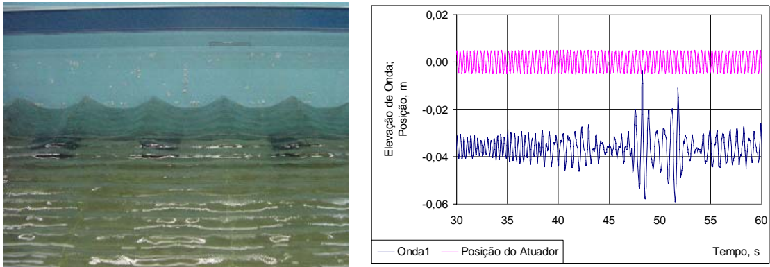
Figura 8 – Ilustração da ocorrência de ressonância transversal
