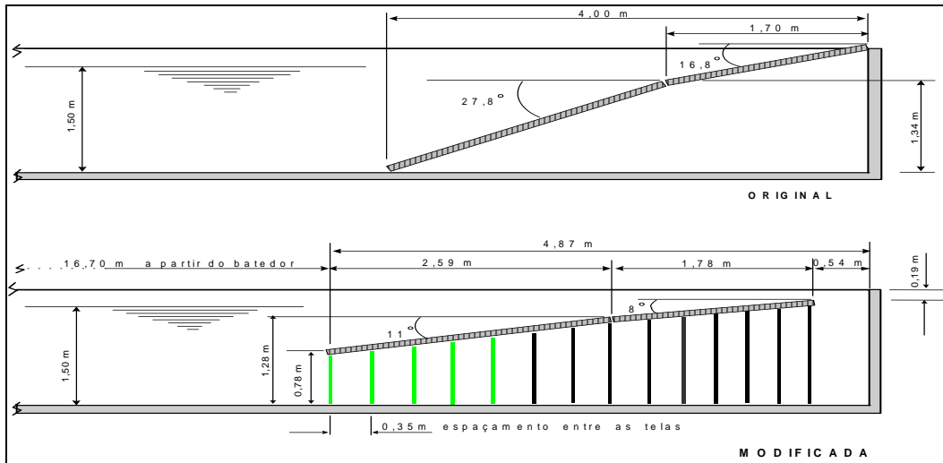
Figura 1 - Croquis das configurações do absorvedor de energia de onda.
